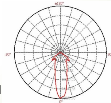
R1光形圖
